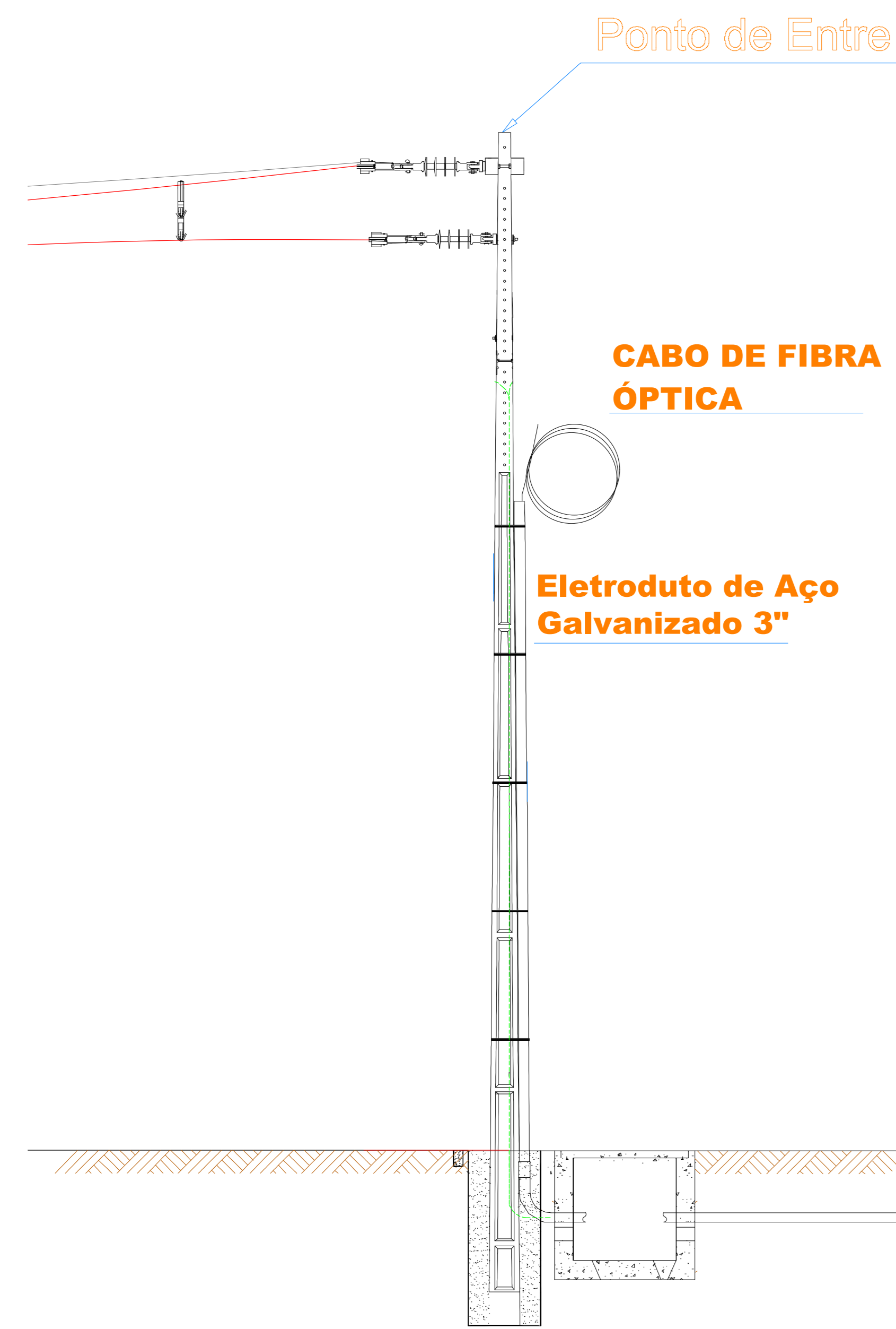
DETALHE 01 - ENTRADA DE FIBRA ÓPTICA LOCALIZADA NA ENTRADA DE ENERGIA ESCALA SEM ESCALA
