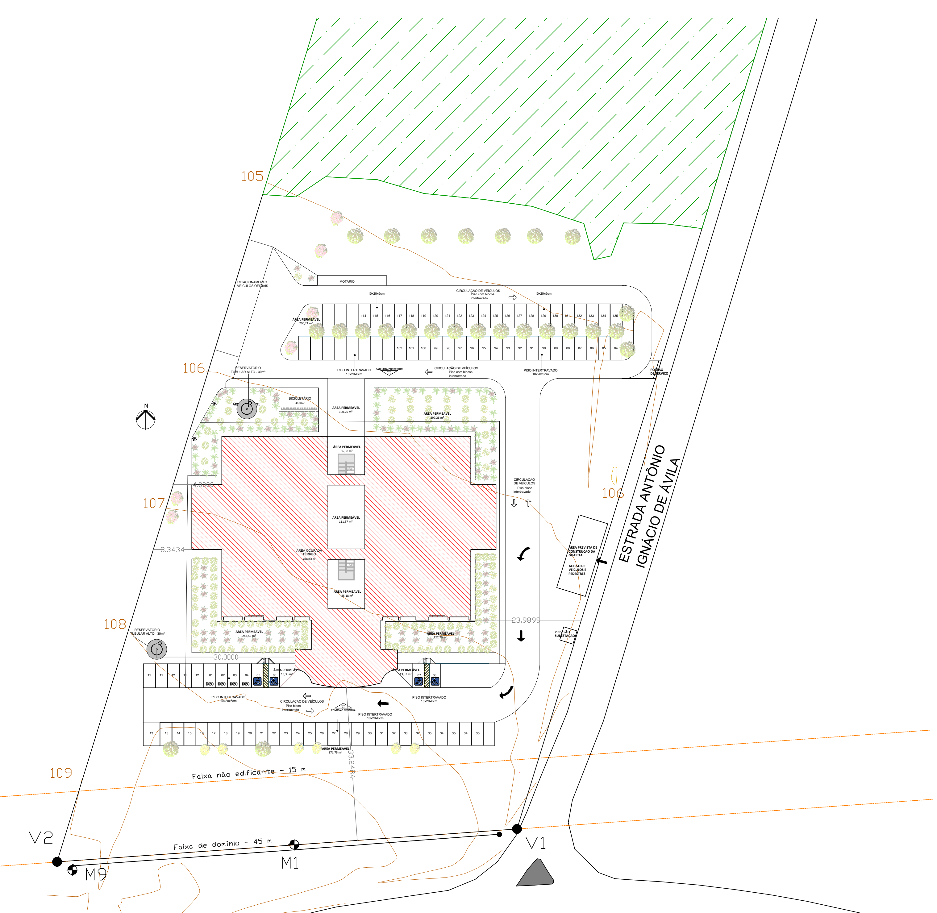
PLANTA DE ACESSO DAS VIATURAS Escala / 1:500
